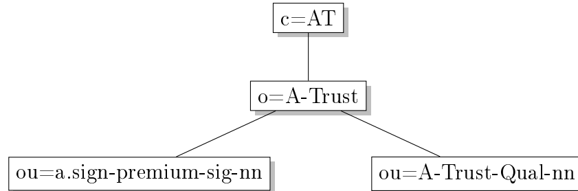
Abbildung 2: A-Trust Verzeichnisbaum
