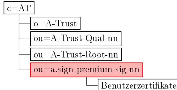
Abbildung 2: A-Trust Verzeichnisbaum
