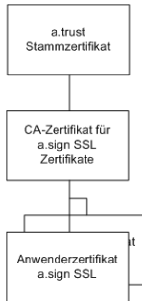
Abbildung 2: Zertifizierungshierarchie
